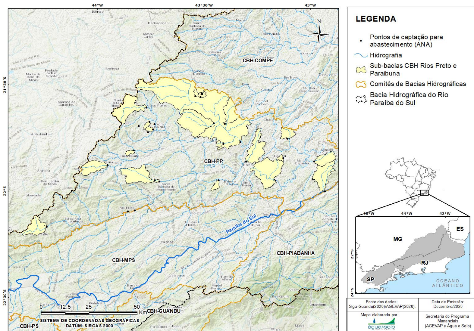
Figura 2.2 - Localização das sub-bacias do CBH Rios Preto e Paraíba
